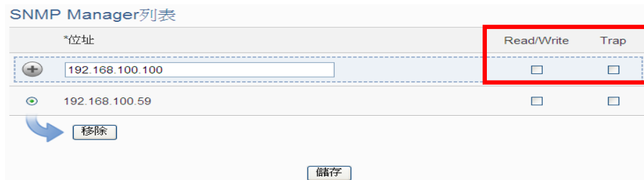
图 5-13: SNMP Manager 的工作模式设定
