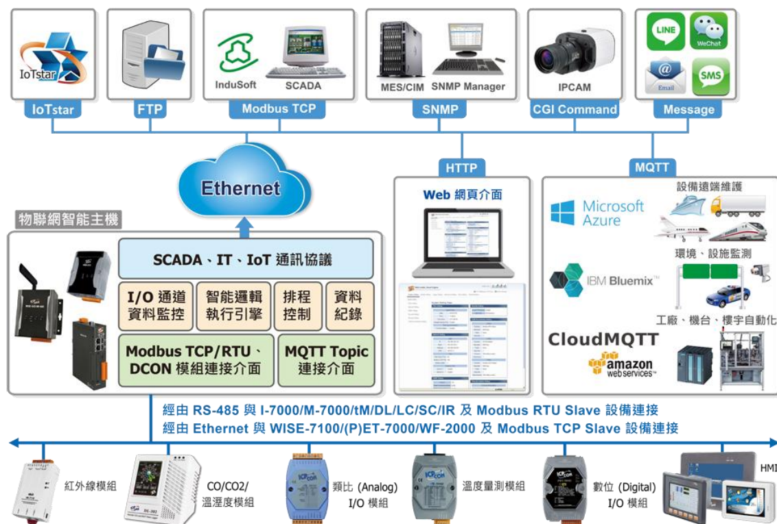
圖 1-1 : WISE-523x/WISE-224x 系統架構圖
