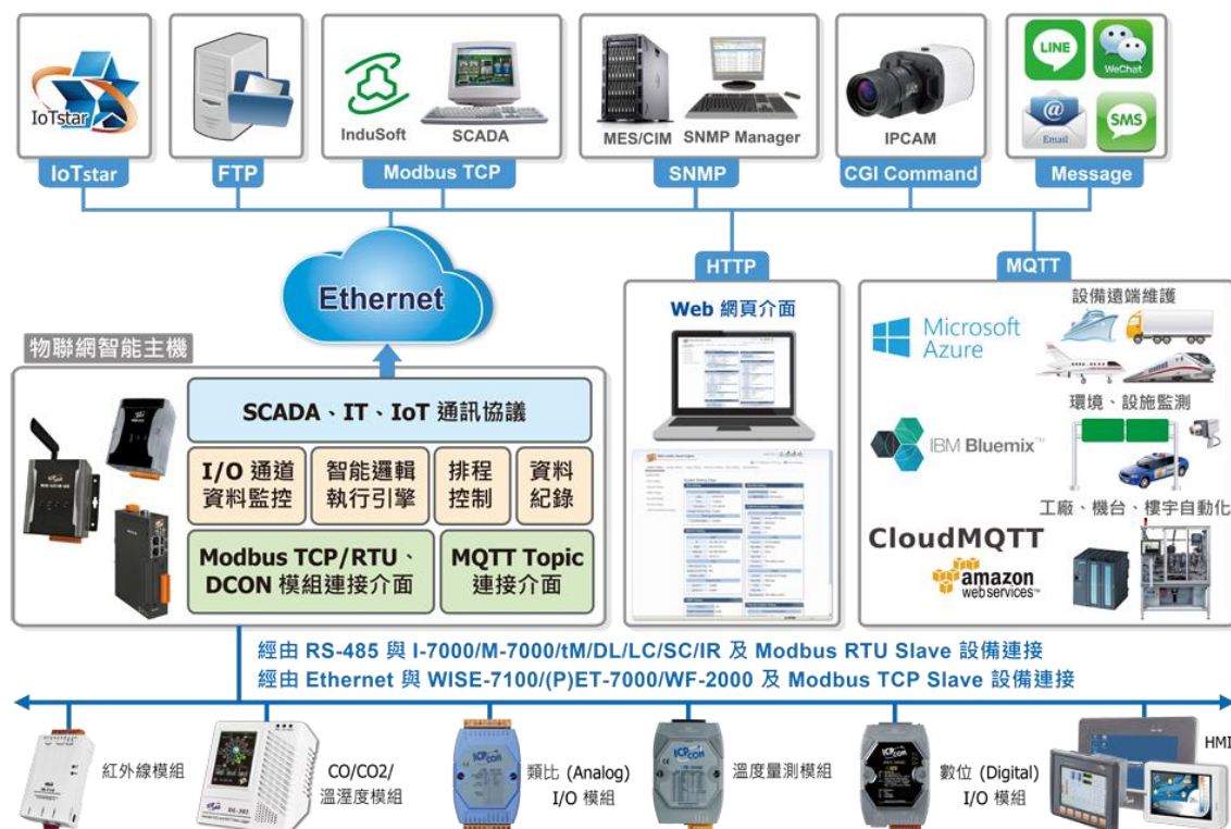
图 1-1: WISE-523x/WISE-224x 系统架构图
