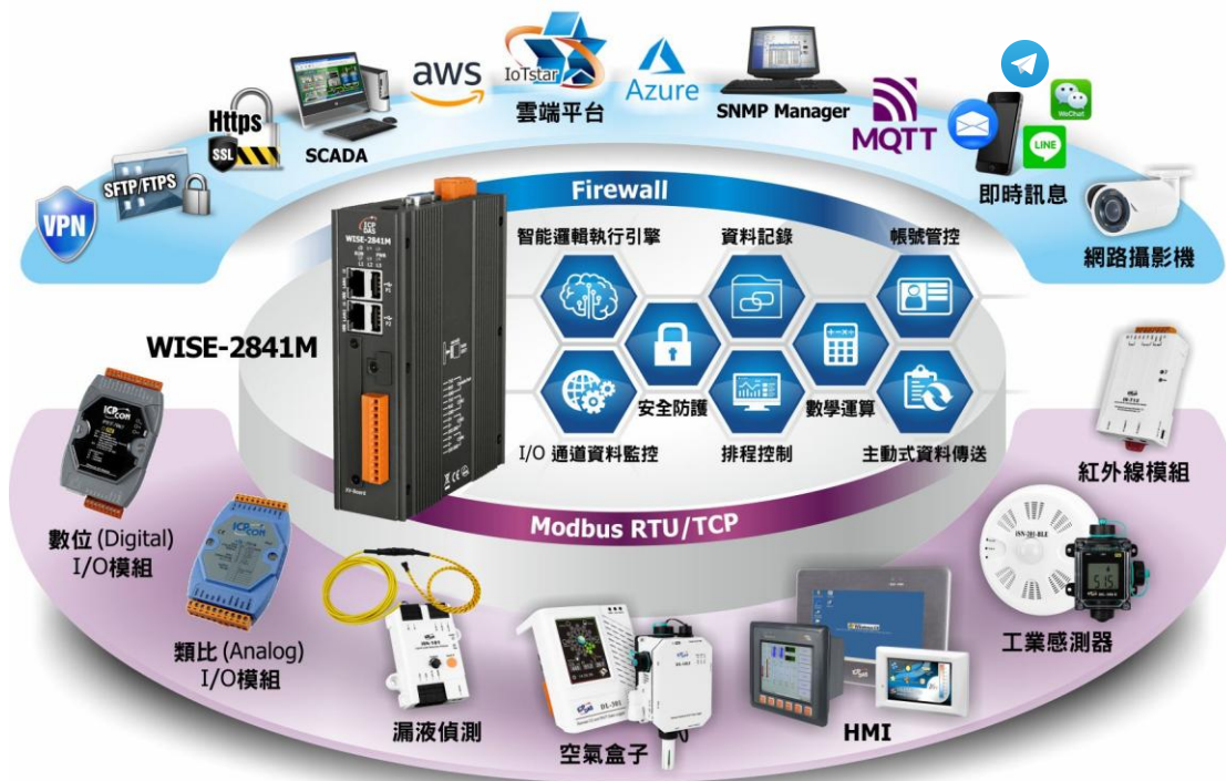
圖 1-1：WISE-2841M 系統架構圖
